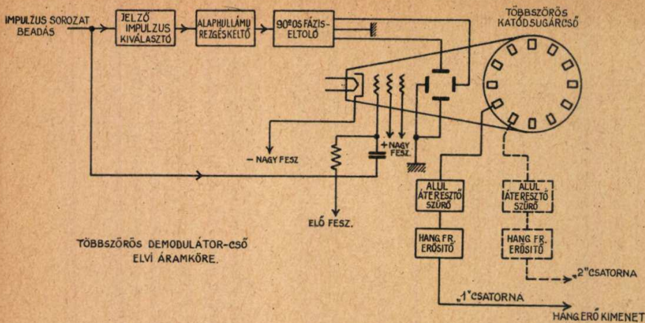
3) ábra. Impulzus-idő moduláció.
