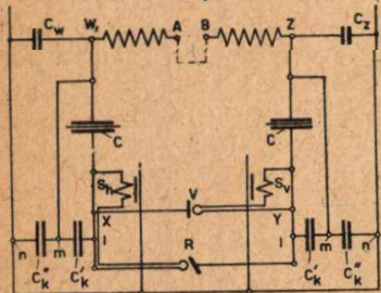
9 és 9a ábra Egy Claassen szerint módosított Villard kapcsolású gép
