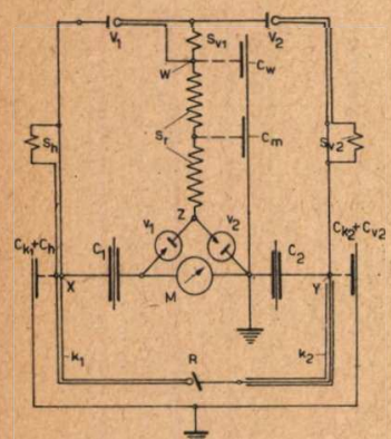
10 ábra. Egy Liebnow-Greinacher kapcsolású gép magasfeszültségi köre
