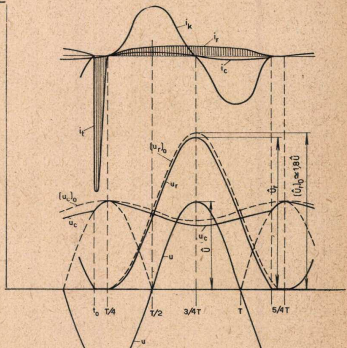
⑧ ábra. A Villard-kapcsolású gép magasfeszültségű körében fellépő feszültségek és áramok. Feltételek: C = 4000 cm, C_k = 500 cm; n = 50 Hz, \hat{U} = 200 kV, i_r = 2 mA. a) (u_c)_0 = a két C -kondenzátor összefeszültségének pillanatnyi értéke, a gép üresjáratánál, u_c = ugyanaz a gép megterhelésénél. (u_r)_0 = gép-feszültség az üresjáratban, u_r ugyanaz a gép megterhelésénél. b) A röntgentranszformátor szekundér tekercsén át haladnak: 1. i_i = a C -kondenzátorok töltési árama; ennek összarmennyisége azonos azzal az árammennyiséggel, amely a T/4 \dots T + t_0 időszakban a röntgensövön halad át. 2. i_c = a röntgentranszformátor kapacitási árama (sarkkondenzátorok C_1 = C_2 = C_3 ). 3. i_k = a kábelek töltési és kiszülési árama.
