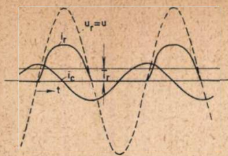
3) ábra. A 2-ik ábrában feltüntetett árammérőn át haladó áramok görbéi. i_r = a röntgensővön áram; i_c = ezen áram aritmetikai középértéke; i_e = a röntgentranszformátor, a fűtőtranszformátor és a kábelek eredő kapacitási árama.
