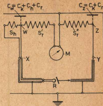
② ábra. Egy egyszerű félhullámú gép magas feszültségű köre. 1
