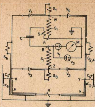
4) ábra. Egy négy szelepes diagnosztikai röntgengép magasfeszültségű köre egy beléje kapcsolt (M-v_1-v_2) -árammérő berendezéssel és egy Ockenden-léle terciér körrrel.
