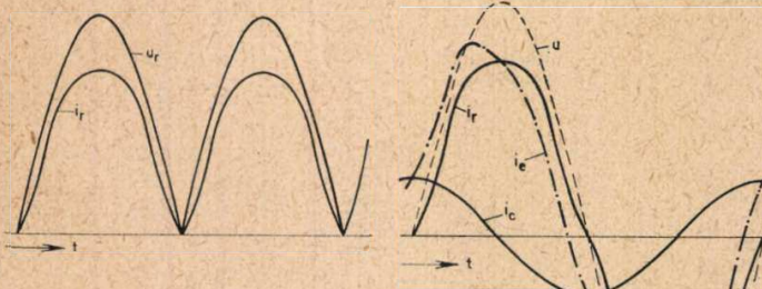
5) ábra. A négy szelepes gép magasfeszültségű körének két különböző helyén haladó áramok. Felvételi üzem; az u_r gépészültség görbéje gyakorlatilag azonos az egyenirányított u feszültség görbéjével.
