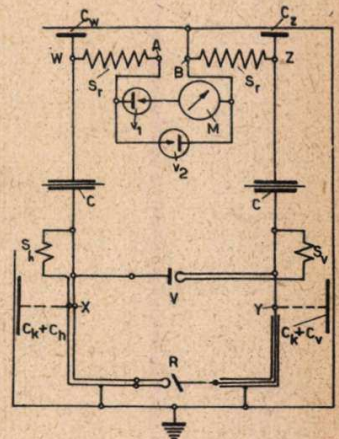
⑥ ábra. A négyfázisú gép magasfeszültségű körének két helyén haladó áramok. Feltételek: minden egyes kábel hossza = 4 m; átvilágítási üzem; n = 50 Hz, U_r = 80 kV, i_r = 2 mA. — A kábelek minden félperiódus első felében az \hat{U}_r értékre feltöltődnek; a T/4 pillanatban oly nagy töltéssel rendelkeznek, hogy a csak 2 mA-t fogyasztó röntgensövet 3/4 T -én át táplálhatnának. Erre ugyan nem kerül sor, mert a (T/2 + t_0) — pillanatban a röntgentranszformátortól szolgáltatott feszültség az időközben félig kimerült kábelek feszültségén felülkerekedik; a kábelek kiszülése fennakad és újra töltődnek. Az u_r feszültség ez esetben nem \hat{U}_r és 0 , hanem \hat{U}_r és (U_r)_{\min} között lüktet. a) i_r = a röntgensöv árama; ezt a t_0 \dots T/4 időközben ( i_r = i_r' ) a röntgentranszformátor szolgáltatja, a T/4 \dots (T/2 + t_0) — időszakban azonban ( i_r = i_r'' ) a kábelpár. A röntgensövön félperiódusonként áthaladó árammennyiség = q_1 + q_2 . b) A röntgentranszformátor szekundér tekercsén át folyik: 1. a röntgentranszformátor részéről a t_0 \dots T/4 időszakban szolgáltatott i_r' csőáram (ennek mennyisége = q_1 ). 2. a kábelek i_k' töltőárama (a kábelekbe ömlő egész árammennyiség azonos nagyságú az i_k'' -nek a) alatt sraffirozás által feltüntetett időintegráljával, tehát = q_2 -vel), 3. az S_1 , S_2 és S_3 tekercsek i_c kapacitási árama. Az M -en félperiódusonként áthaladó árammennyiség ugyancsak = q_1 + q_2
