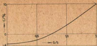
① ábra. Egy árammennyiségmérő korrekciógörbéje.
