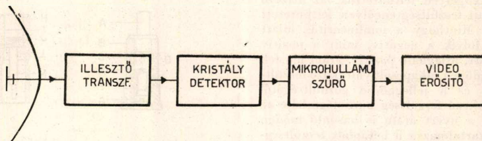
1. ábra. Kristálydetektoros vevőkészülék elvi felépítése
