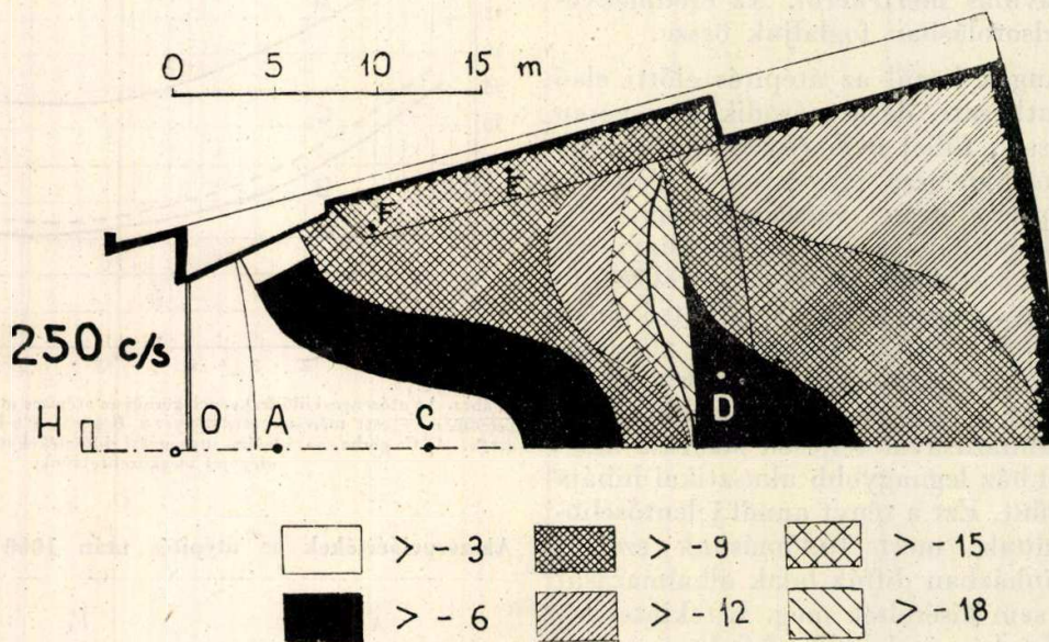
10. ábra. A hangnyomás eloszlása átépítés után 250 c/s frekvencián. A hangszórók H helyben állnak, a 0-dB szint O-ban mérhető. A, C, D, E és F utóhangidő mérési helyek.
