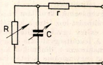
5. ábra. Kristályegyenirányító helyettesítő áramköre
