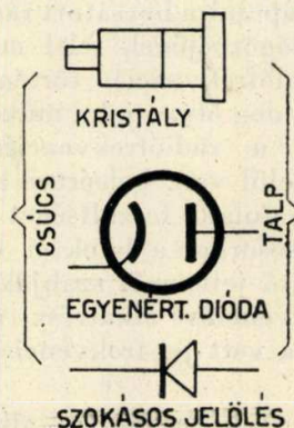
4. ábra. Kristályegyenirányított szerelvénnyel polaritása
