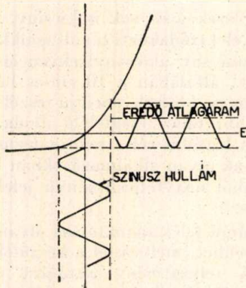
2. ábra. A detektor működése.
