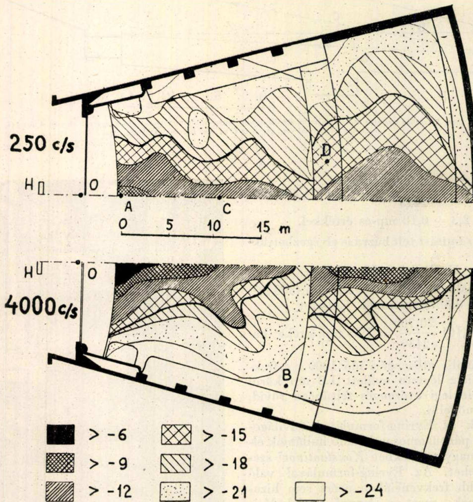
7/a ábra (felső kép) A hangnyomás eloszlása átépítés előtt 250 c/s frekvencián. A hangszórók H helyen állnak, a 0-dB szint O -ban mérhető. A , C és D helyek az utózenngési idő mérőhelyei.
