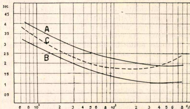
6. ábra. Az utózungési idő frekvenciagörbéi az átépítés előtt. Az A görbe az üres teremben végzett mérések eredménye, a B görbe a telt teremre átszámított érték. A C görbe az ideális utózungési időértékeket szemlélteti.
