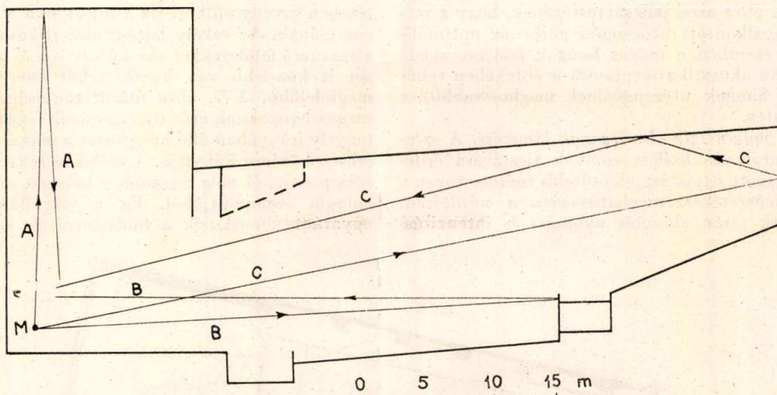
4. ábra. A színház vázlatos metszetrája az átépítés utáni proszcénium-mennyezettel (szaggatott vonal). A felvevő mikrofon M helyen van, A , B és C az első három visszhang útja.
