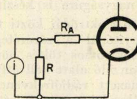
6. ábra. A kristálydetektoros vevő modulálófrekvenciánál működő áramköre
