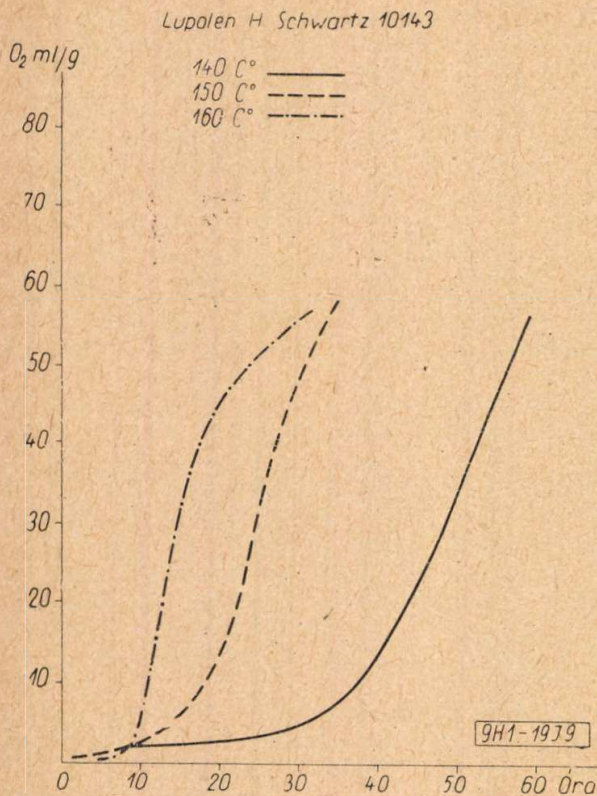
9. ábra Lupolen H Schwartz 10413
