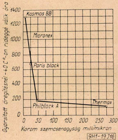
16. ábra A korom szemcsenagyságának hatása a polietilén gyorsított öregítésére. (Ind. Eng. Chem. 42. 1950. 2322)
