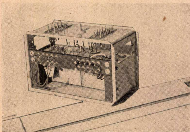
14. ábra. Modulátor-demodulátor laboratóriumi modellje
