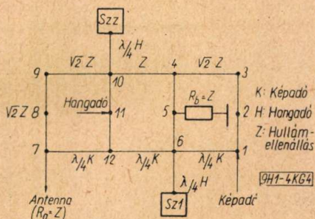
4. ábra. A keverősűrű elve
