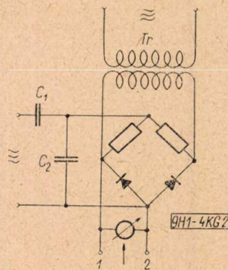
2. ábra. A reflektométer elve
