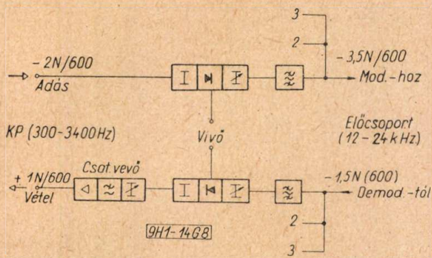
8. ábra. 3-csatornás előcsoporthoz tartozó csatornamodulációja
