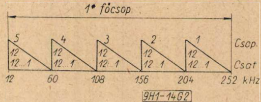
2. ábra. 60-csatornás rendszer szimmetrikus kábelérpárra ajánlott frekvenciakiosztása
