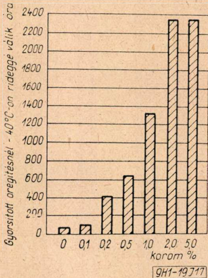
17. ábra A korom töménységének hatása a polietilén gyorsított öregítésére. (Ind. Eng. Chem. 42. 1950. 2323)
