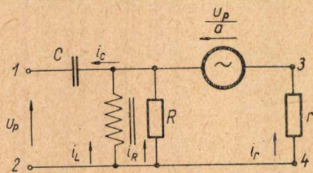
2. ábra. Q : a fojtó vaskeresztmetszete, w : a fojtó menet száma, l : a fojtó erővonal hossza, B : a fojtó indukciója, H : a fojtó mágneses térerere, a : a hálózati transzformátor menetszám áttétele
