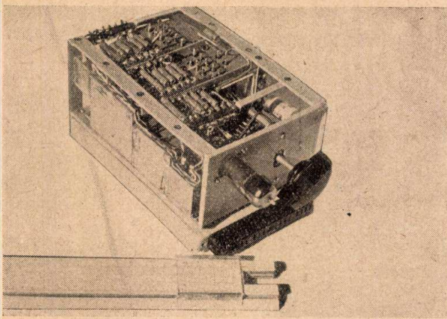
13. ábra Csatorna vevő laboratóriumi modellje
