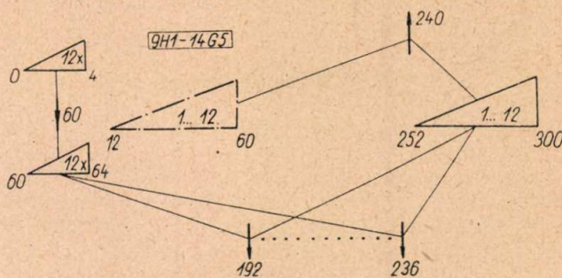
5. ábra. Nagyfrekvenciás előmoduláció
