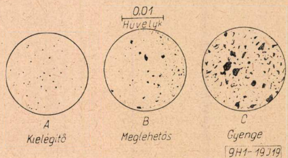
19. ábra A korom elosztásának hatása a polietilén gyorsított öregítésére. (Ind. Eng. Chem. 42. 1950. 2324)
