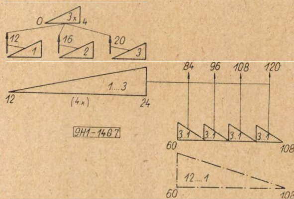
7. ábra. Előcsoport moduláció
