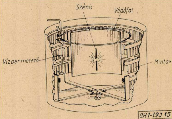
15. ábra Átalakított Weather-Ometer. (Ind. Eng. Chem. 42. 1950. 2321)
