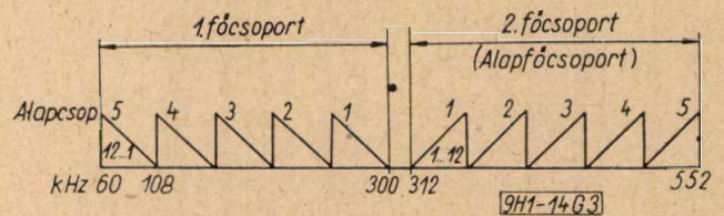
3. ábra. CCITT alapfőszoport
