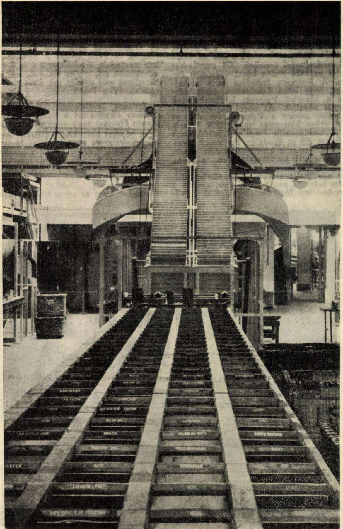
2. ábra. Mount Pleasant postahivatal irányító berendezése nagyobb terjedelmű levélpostai küldemények szétosztására.
