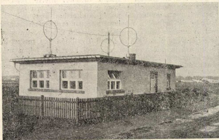
8. ábra: „Repülőtéri iránymérő állomás szokásos kivitelben.” (Telefunken felvétel.)
