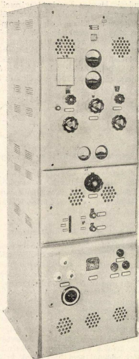
13. ábra: „200 wattos középhullámú adó.” (Telefunken felvétel.)
