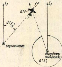
7. ábra: „Helymeghatározás keresztméréssel.”
