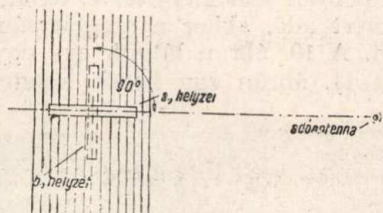
9. ábra. „A keretantennával való iránymeghatározás elve.”
