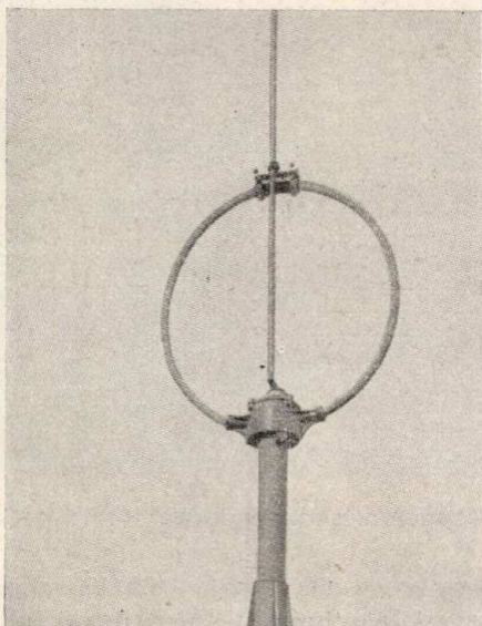
10. ábra: „Egyszerű keretantenna a segédantennával.” (Telefunken felvétel.)
