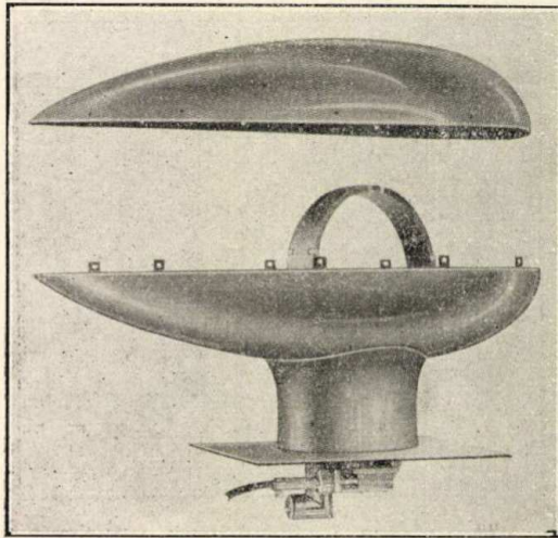
2/b. ábra: „Áramvonalas burokkal körülvevett repülőgép keretantenna.” (Marconi felvétel.)
