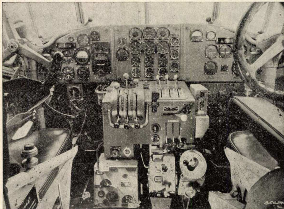
1. ábra: „Ju. 52. típusú utasszállító repülőgép műszerei és rádió berendezése.” (Junkers felvétel.)
