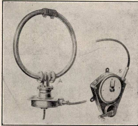
2/a. ábra: „Keretantenna repülőgéphez.” (Marconi felvétel.)
