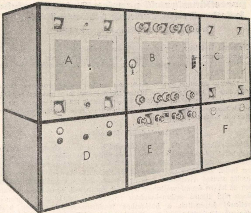
14. ábra: „1,5 kilowattos középhullámú adó.” (Marconi felvétel.)
