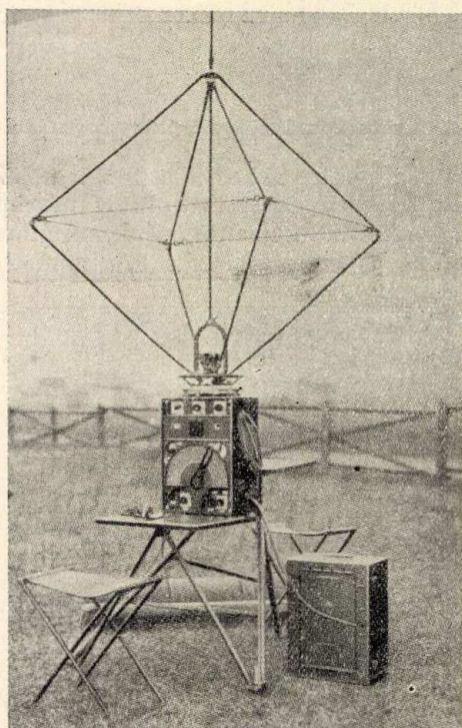
11. ábra: „Kettős keretantenna segédantennával” (Telefunken felvétel.) Telefunken
