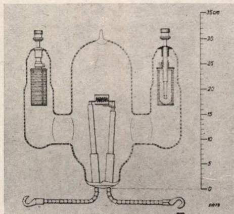
6. ábra: Kétanódos gáztöltésű egyenirányítócső (250 volt 40 Amper egyenáramra.)
