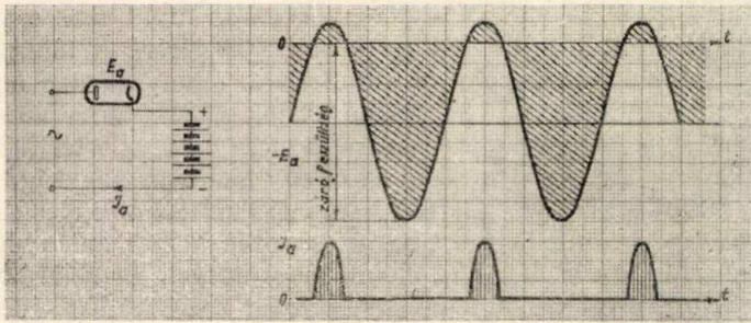
2. ábra: Ellenfeszültséggel dolgozó egyenirányító kapcsolás anódáram és anódfeszültség görbéi.
