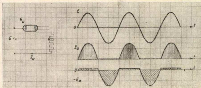
1. ábra: Ohmikus terhelésre dolgozó egyfázisú egyenirányító áram- és feszültségviszonyai.
