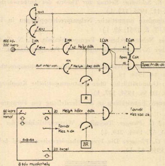
1. ábra. Nyíregyházi aut. távb. közp. kapcsolási vázlata.
