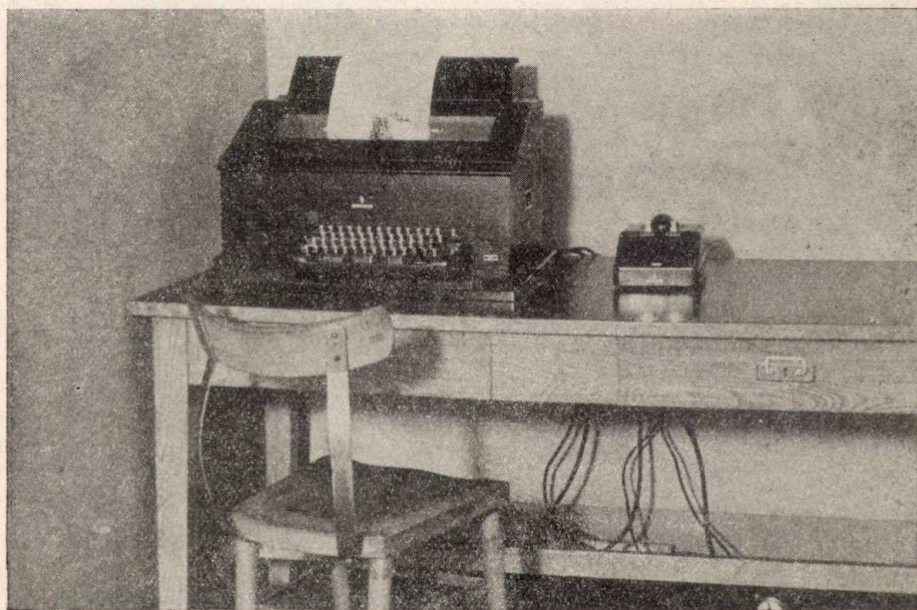
Előfizetői távgépirókészülék.
