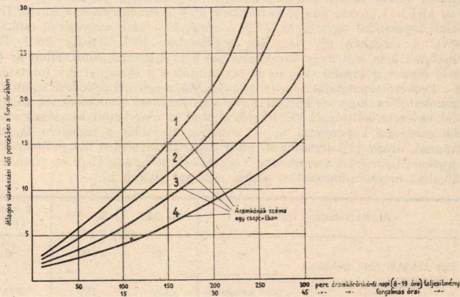
Áramkörök kihasználása a várakozási idő és a csoport-nagyság függvényében.
