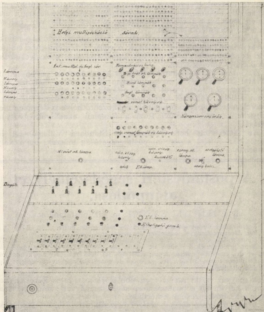
3. ábra. A szombathelyi interurbán kapcsolószekrény elrendezése.
